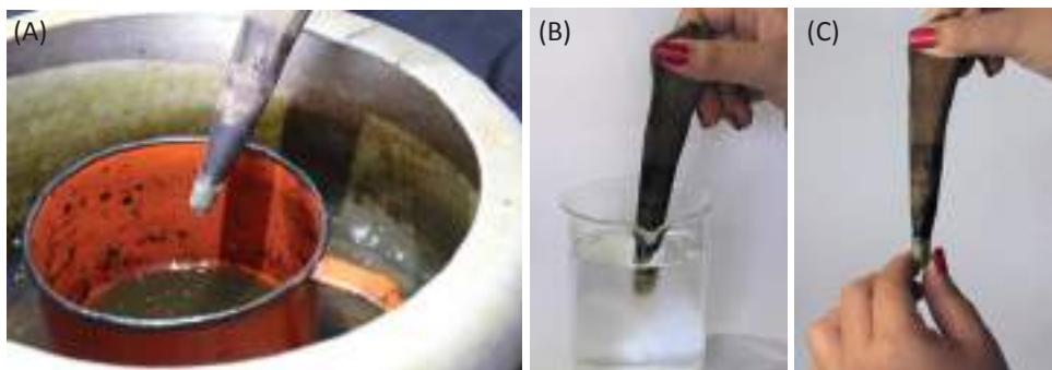
Figura 23. Modelagem de cúpulas de cera; (a) Bastonete é mergulhado por duas a três vezes na cera liquefeita; (b) Bastonete é mergulhado na água para a solidificação da cera; (c) A cúpula moldada é retirada do bastonete por meio da torção desta
