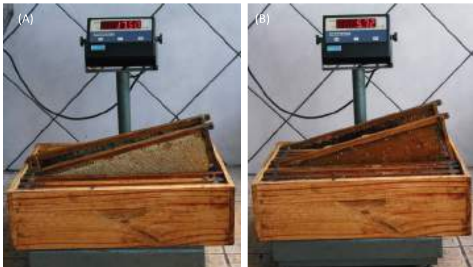
Figura 6. Avaliação da produtividade de mel. (a) Pesagem das melgueiras cheias (antes da centrifugação); (b) Pesagem das melgueiras vazias (após a centrifugação)
