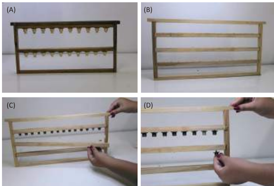
Figura 9. Modelos de sarrafo porta cúpula. (a) Quadro porta cúpulas adaptado a partir de um caixilho de ninho padrão Langstroth com sarrafo de 3,5cm de largura; (b) Quadro porta-cúpulas estreito com sarrafos de 1,5cm de largura, removíveis (c) sarrafos porta-cúpulas removíveis e (d) fixação das cúpulas modelo JzBz® no sarrafo
