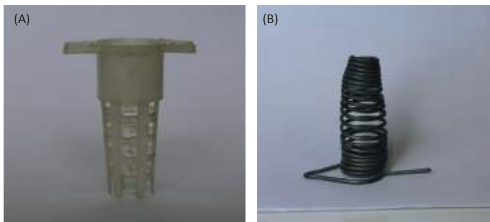
Figura 19. Introdução de realeiras. (a) Protetores tipo West confeccionado em plástico; (b) Protetores tipo West confeccionado com arame em espiral
