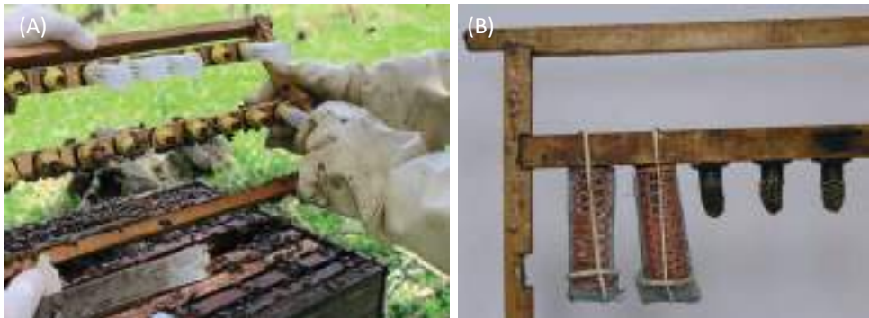
Figura 22. Engaiolamento das realeiras para nascimento em colmeia recria. (a) Adaptação de gaiolas para o nascimento das rainhas na colmeia recria; (b) Gaiolas adaptadas a partir de bob de cabelo
