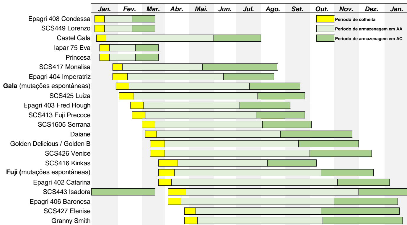
Figura 1. Período de colheita e período potencial de comercialização para maçãs armazenadas em atmosfera do ar (AA, O_2 = 21\% ) ou atmosfera controlada (AC, O_2 < 1,0\% ), a 0,8^\circ C .
